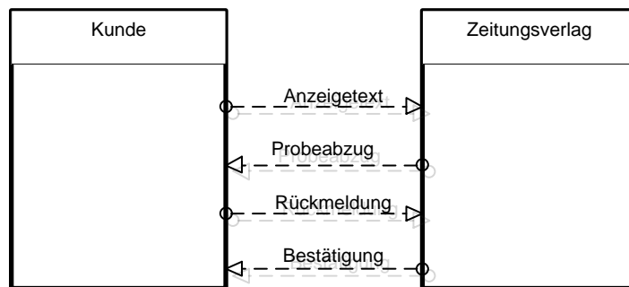
Abbildung 39 Beispielhafter Nachrichtenaustausch
