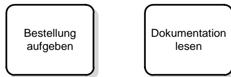
Abbildung 5 Tasks
