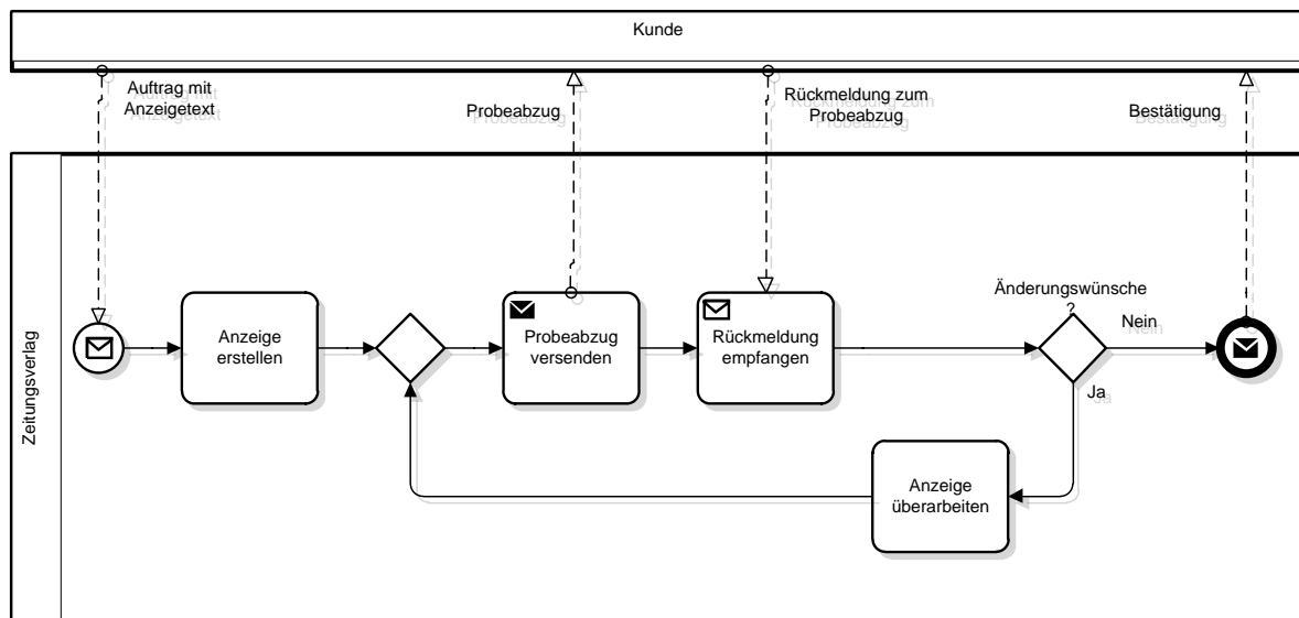
Abbildung 25 Öffentlicher Prozess
